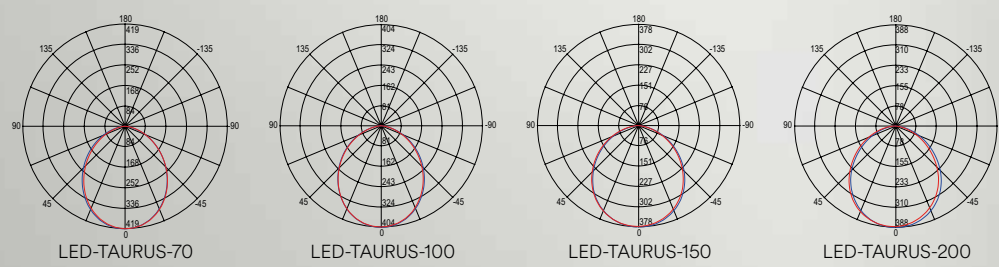
Fotometria del prodotto / Photometric curve
